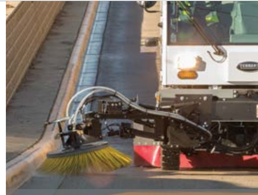
OPTIONAL VARIO SWEEPING BRUSH™
